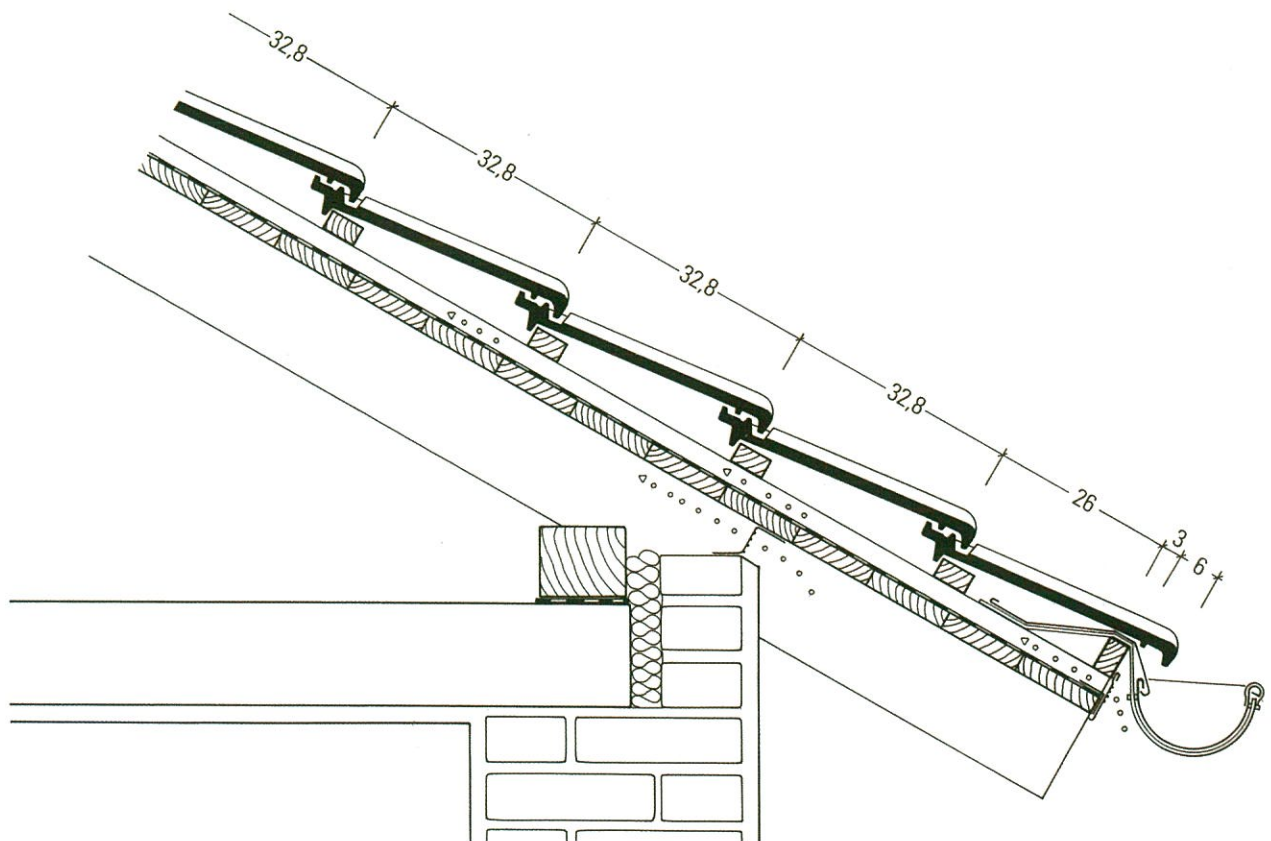
مقطع يوضح طريقة تركيب القرميد أعلى السقف Section shows the way of fixing Roofing-tiles on the roof
