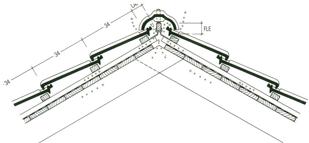
مقطع يوضح طريقة تركيب القرميد أعلى السقف Section shows the way of fixing Roofing-tiles on the roof
