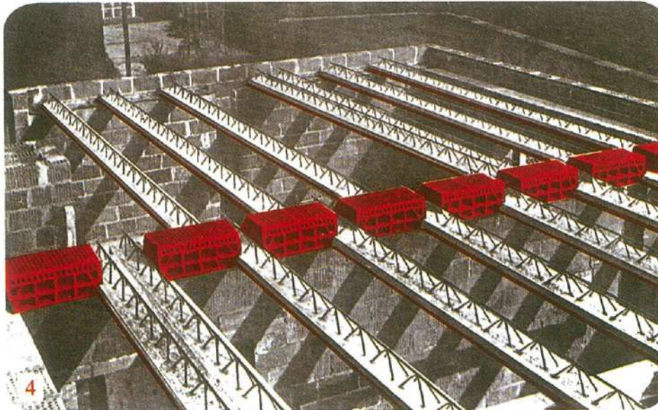
٣، ٤- بعد وضع هذه الجسور مسبقة الصنع يتم تركيب تلك الهوردي بوقت قصير جداً .
