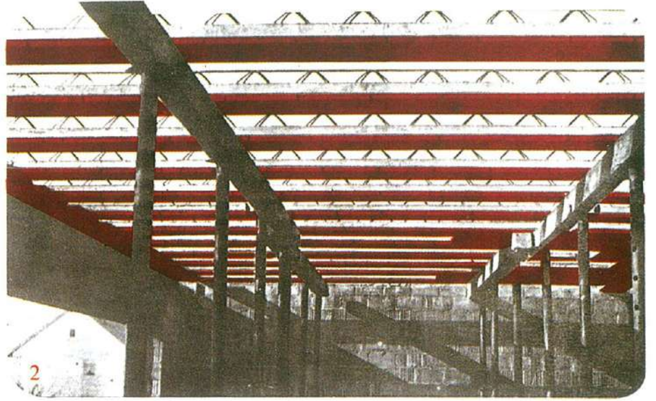
٢- هذه الغرفة الكبيرة تحتاج فقط إلى عدد ٢ دعامة افقية لحمل الجسور خلال أعمال صب السقف والتي تزال بعد أن تصل الخرسانات إلى القوة المطلوبة .
