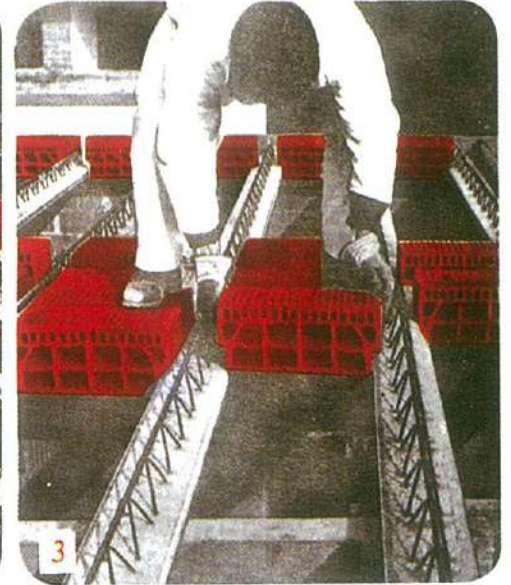
٣، ٤- بعد وضع هذه الجسور مسبقة الصنع يتم تركيب تلك الهوردي بوقت قصير جداً .
